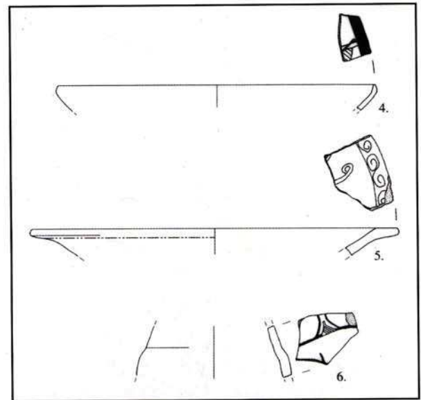
Çizim 2: Evreşe-Çokal Köyü Kokarpınar Mevki. Kat. Nr. 4-6. Ölçü 1:3.
