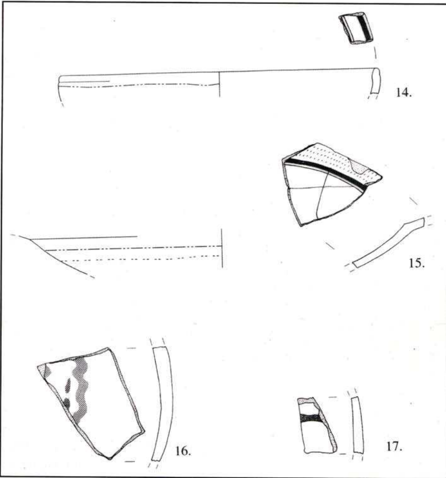
Çizim 5: Evreşe-Kalealtı Köyü, Kat. Nr. 14-17, (Ölçü 1:3)
