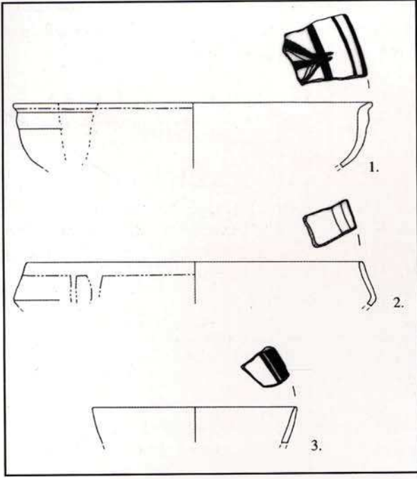
Çizim 1: Evreşe-Çokal Köyü, Kokarpınar mevki, Kat. Nr. 1-3 (Ölçü 1:3).
